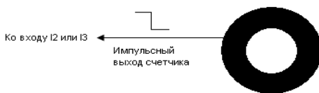
Рис. 14. Подключение импульсного датчика расхода топлива
