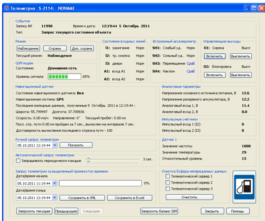
Рис. 39. Окно просмотра текущей телеметрии и управления устройством
