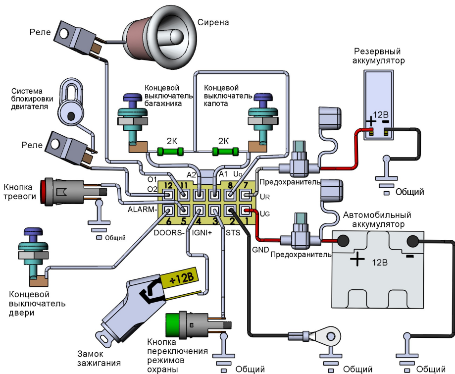
Рис. 32. Схема подключения электропитания, датчиков и исполнительных устройств в конфигурации, предназначенной для охранно-поисковых задач
