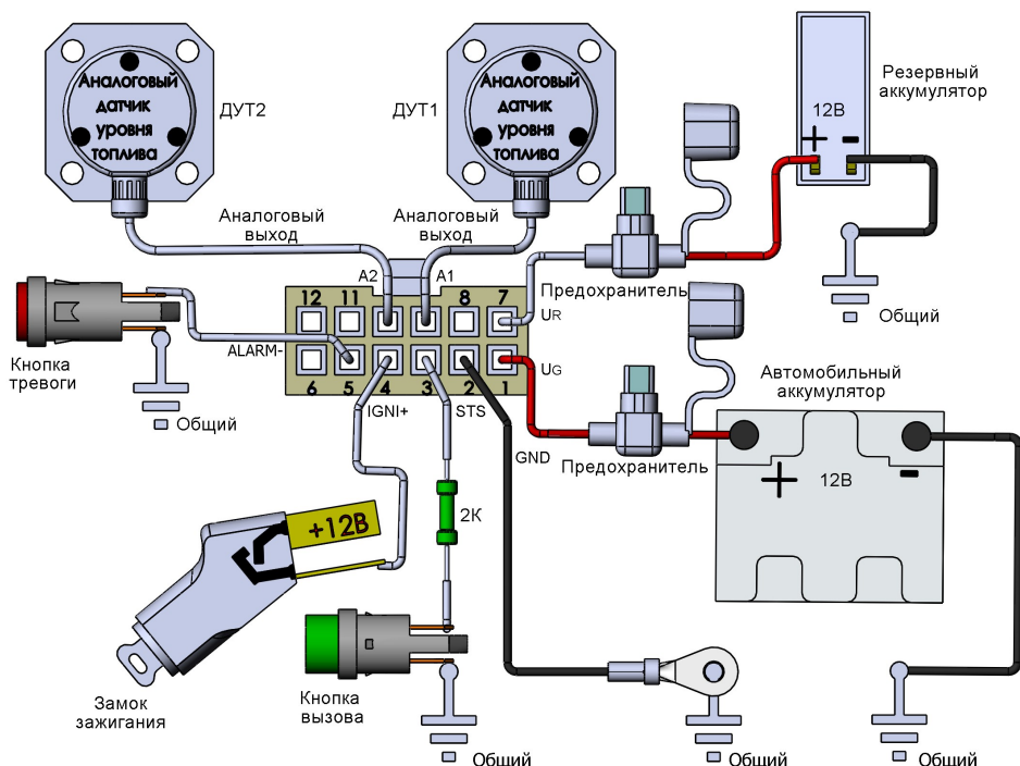
Рис. 30. Схема подключения электропитания, датчиков и исполнительных устройств в конфигурации, предназначенной для мониторинга автотранспорта
