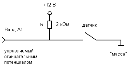
Рис. 19. Схема подключения датчика к А1, замыкающегося на землю
