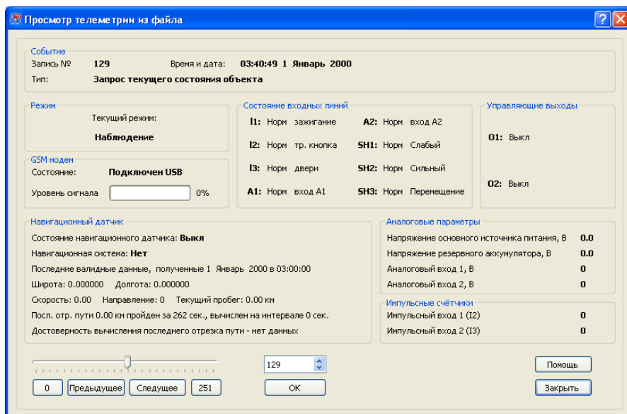
Рис. 41. Окно просмотра телеметрии в постраничном виде
