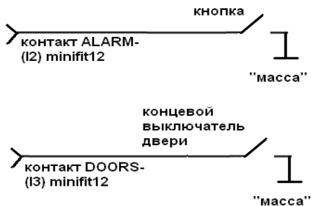
Рис. 12 Подключение сигналов ALARM- и DOORS- для варианта использования входов I2 и I3 с тревожными датчиками
