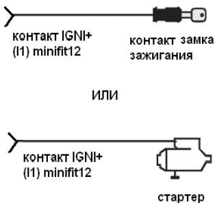
Рис 11. Подключение сигнала от замка зажигания
