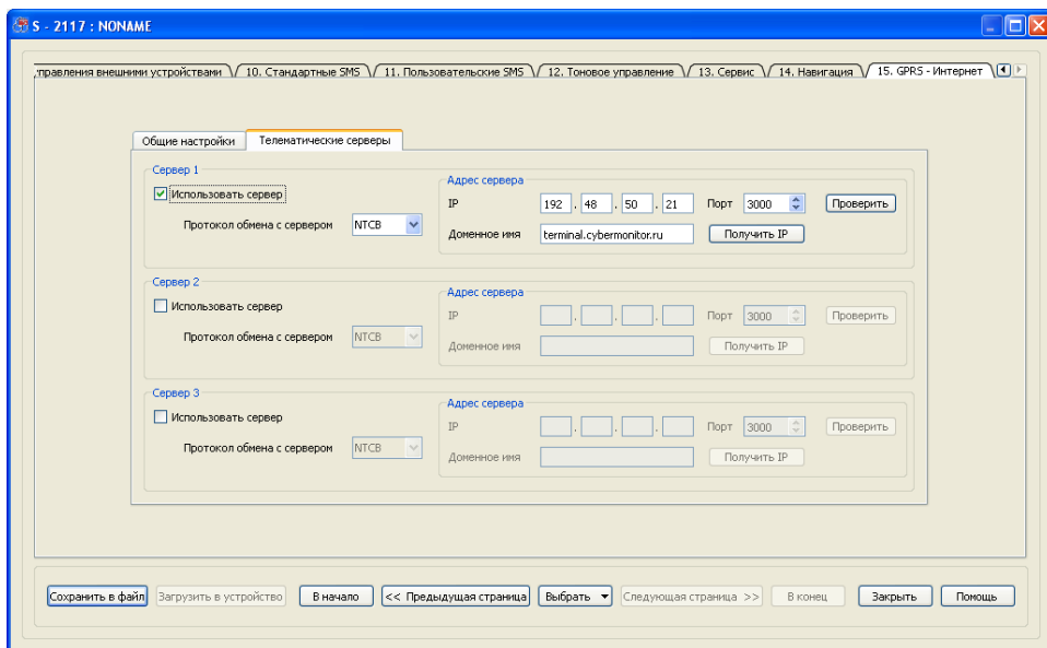
Рис. 55а. Вид вкладки «15. GPRS»
