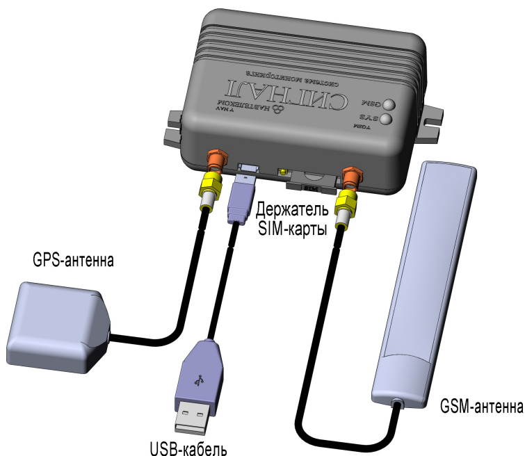
Рис. 29. Схема подключения антенн и установки SIM-карты
