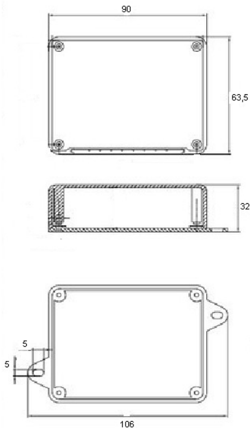
Рис. 33. Установочные размеры системного блока СИГНАЛ (величины указаны в миллиметрах)
