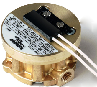
Рис. 13. Импульсный датчик расхода топлива
