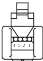
Рис. 28. Схема нумерации контактов на разъеме RJ-11 (вид сверху, если развернуть прибор разъемами антенн к себе)
