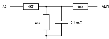
Рис. 22. Принципиальная схема аналогового входа А2
