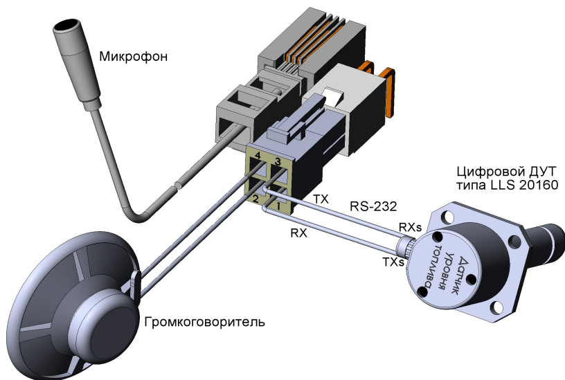
Рис. 31. Схема подключения громкоговорящей связи и цифрового датчика уровня топлива
