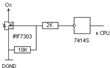
Рис. 24. Принципиальная схема выходов устройства O1, O2 (выходы типа «открытый коллектор»)
