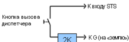
Рис. 26. Схема подключения кнопки вызова диспетчера ко входу STS устройства
