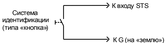
Рис. 25. Схема подключения системы идентификации типа «кнопка» к входу STS устройства
