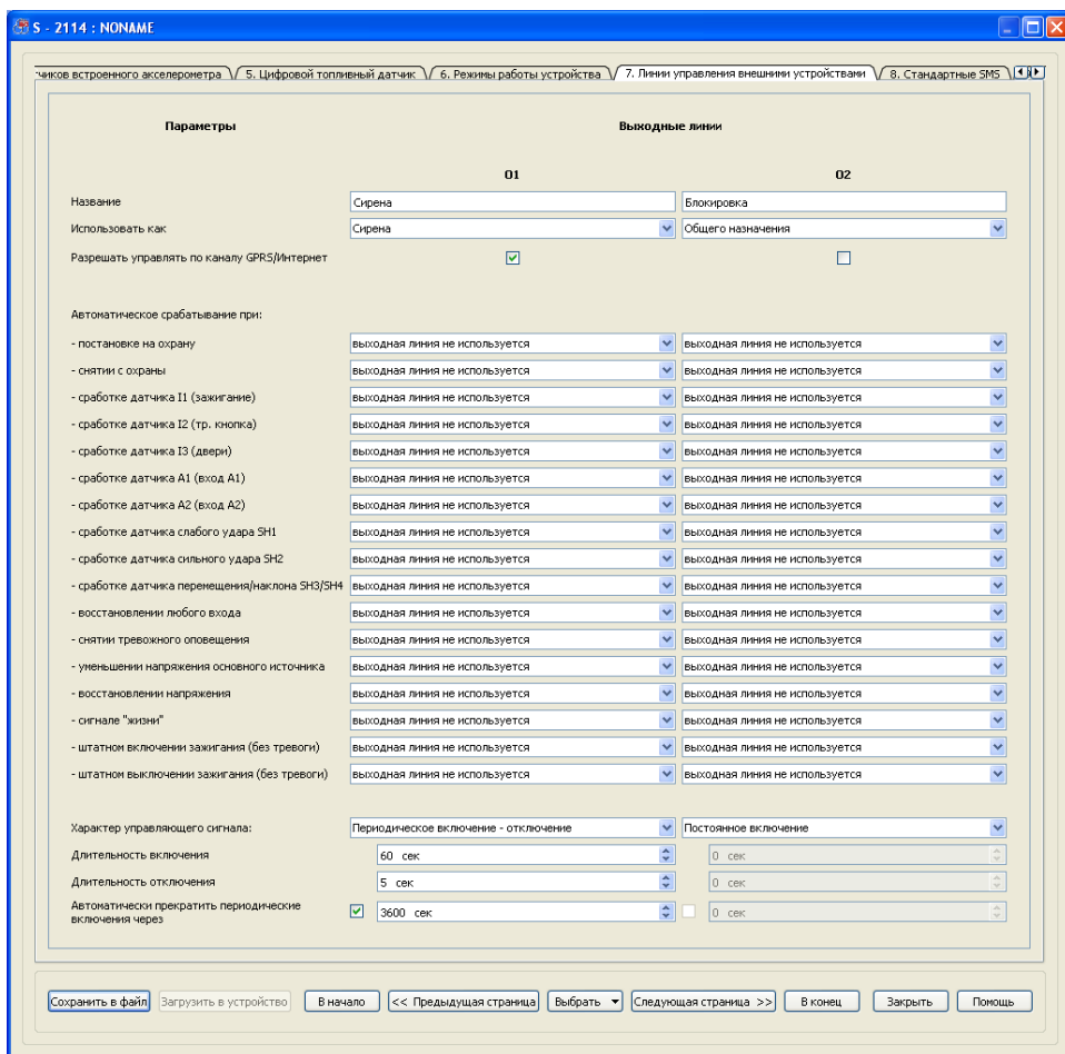
Рис. 49. Вид вкладки «7. Линии управления внешними устройствами»
