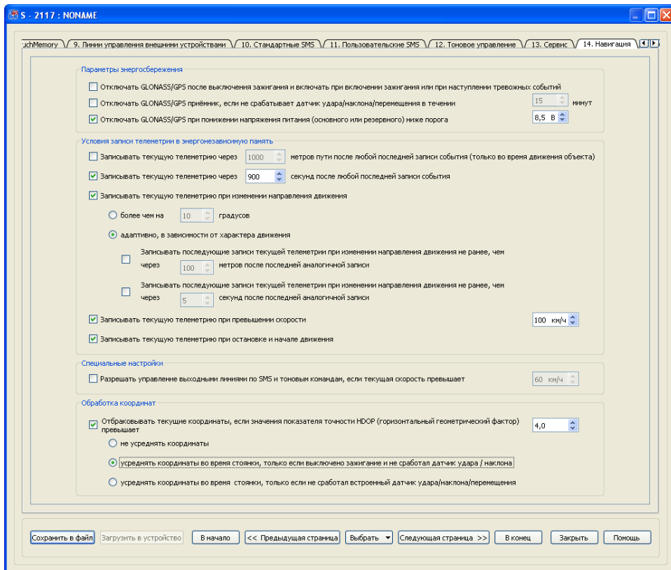
Рис. 54. Вид вкладки «14. Навигация»
