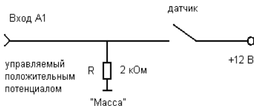
Рис. 20. Схема подключения контактного датчика к А1, коммутирующего положительный потенциал
