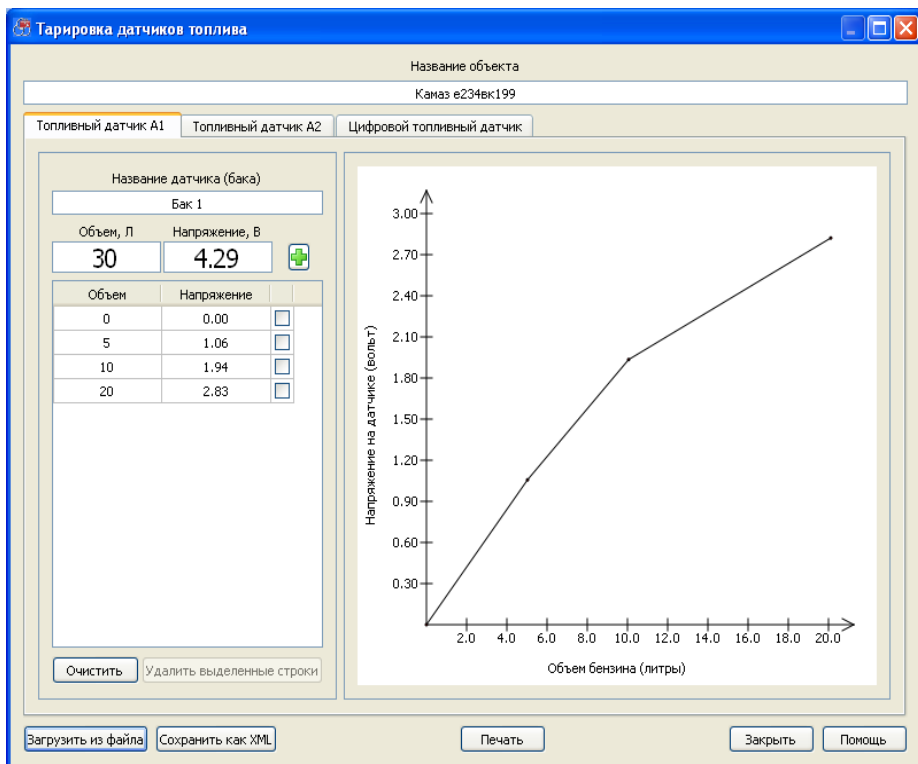
Рис. 57. Вид окна «Тарировка датчиков топлива»
