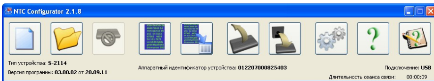
Рис. 35. Главное окно настроечной программы NTC Configurator после подключения устройства
