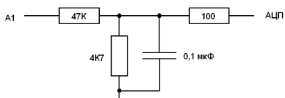
Рис. 21. Принципиальная схема аналогового входа А1
