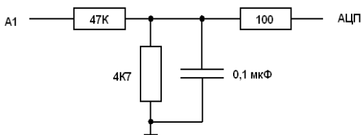
Рис. 20. Принципиальная схема аналоговых входов A1 и A2
