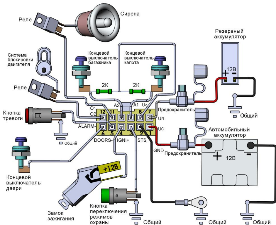
Рис. 27. Схема подключения электропитания, датчиков и исполнительных устройств в конфигурации, предназначенной для охранно-поисковых задач
