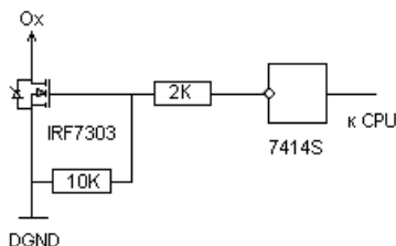
Рис. 22. Принципиальная схема выходов устройства O1, O2 (выходы типа «открытый коллектор»)
