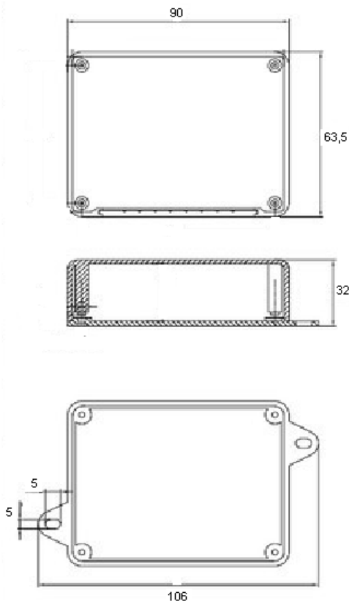
Рис. 28. Установочные размеры системного блока СИГНАЛ (величины указаны в миллиметрах)
