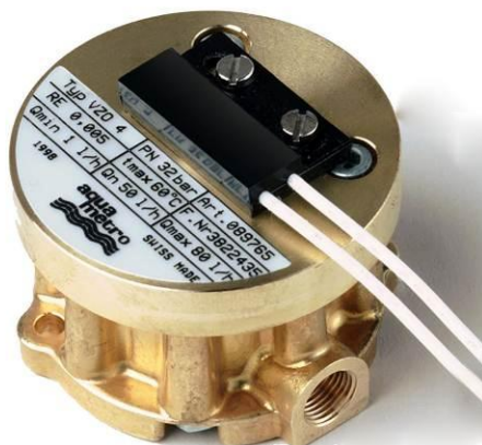
Рис. 12. Импульсный датчик расхода топлива
