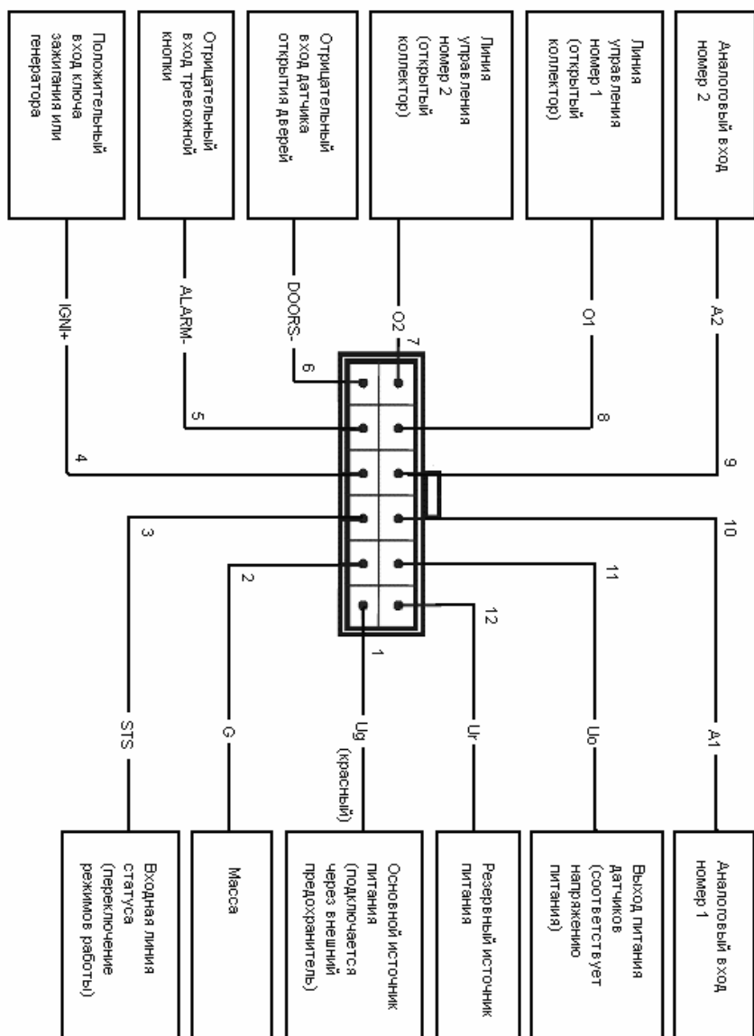
Рис. 9. Подключение 12-ти контактного разъема Minifit
