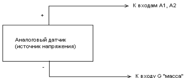
Рис. 15. Схема подключения аналогового датчика к входу I4 или I5
