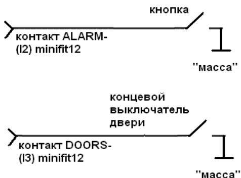
Рис. 11. Подключение сигналов ALARM- и DOORS- для варианта использования входов I2 и I3 с тревожными датчиками
