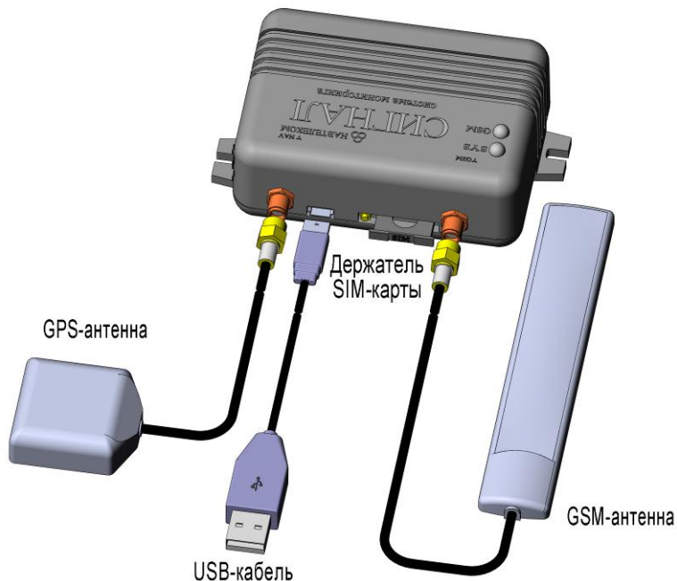
Рис. 25. Схема подключения антенн и установки SIM-карты в устройство СИГНАЛ-2115
