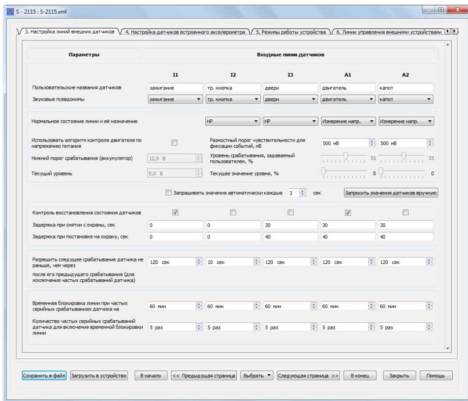
Рис. 55. Вид вкладки «3. Настройка линий внешних датчиков» при подключении ДУТ к линиям А1 и А2
