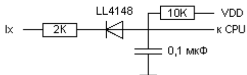
Рис. 14. Принципиальная схема входов I2, I3 устройства
