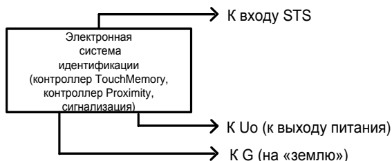
Рис. 24. Схема подключения внешнего контроллера электронной системы идентификации к входу STS устройства
