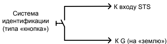
Рис. 23. Схема подключения системы идентификации типа «кнопка» к входу STS устройства
