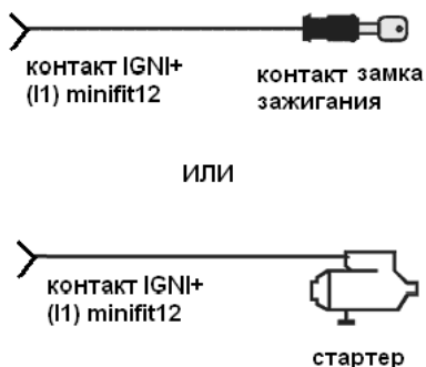
Рис. 10. Подключение сигнала от замка зажигания
