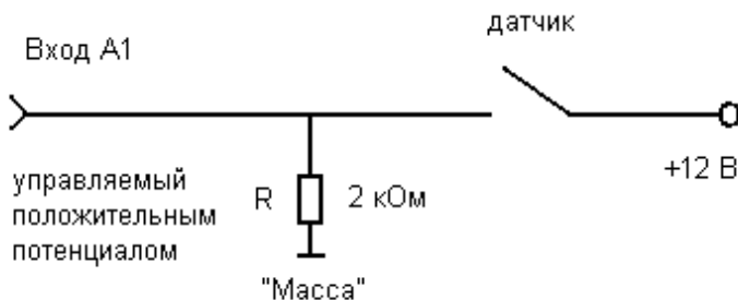
Рис. 18. Схема подключения датчика к A1 и A2, замыкающегося на землю
