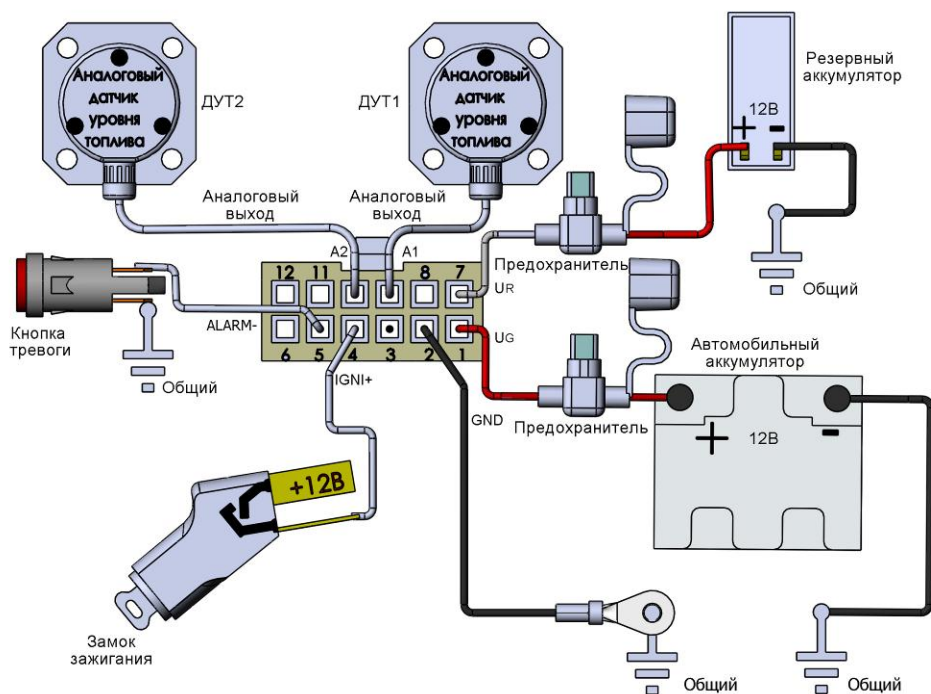
Рис. 26. Схема подключения электропитания, датчиков и исполнительных устройств в конфигурации, предназначенной для мониторинга автотранспорта
