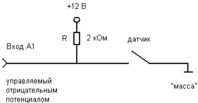
Рис. 19. Схема подключения контактного датчика к A1 и A2, коммутирующего положительный потенциал
