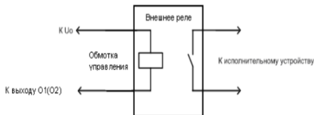
Рис. 21. Схема подключения внешнего реле к выходам устройства O1, O2 (выходы типа «открытый коллектор»)
